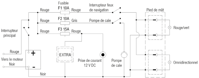
Image 6. Sch.ma de c.blage des mod.les Terhi 450 C/450 Sloep, 450 CC et Terhi 480 TC.
