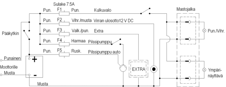
Kuva 9. Terhi Nordic 6020 C -kytentaavaio
