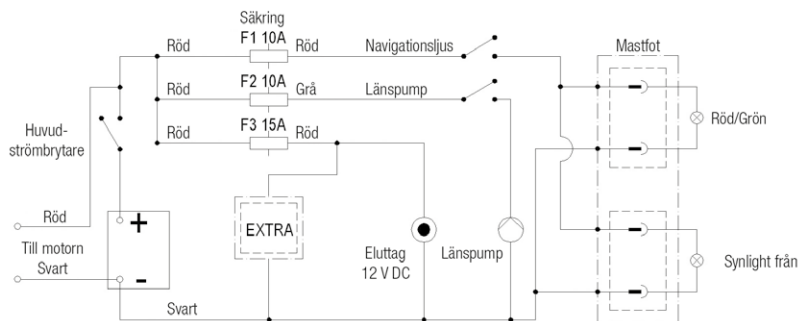
Bild 8. Kopplingschema för Terhi, 450 Sloep, 450 CC, 480 TC, 480 CC och 480 TC.
