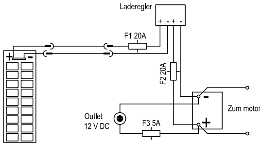
Abb. 12. Schaltplan für Terhi Saiman Solar
