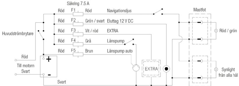
Bild 9. Kopplingsschema för Terhi Nordic 6020 C
