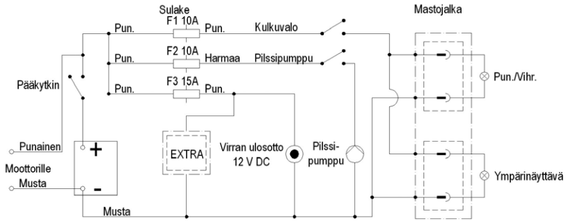
Kuva 8. Terhi 450 SC, 450 Sloep, 450 CC, 450 TC, 480 CC ja 480 TC-kytentaavaio
