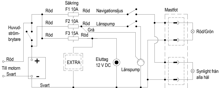
Bild 10. Kopplingsschema för Terhi 480 BR och 480 Sport
