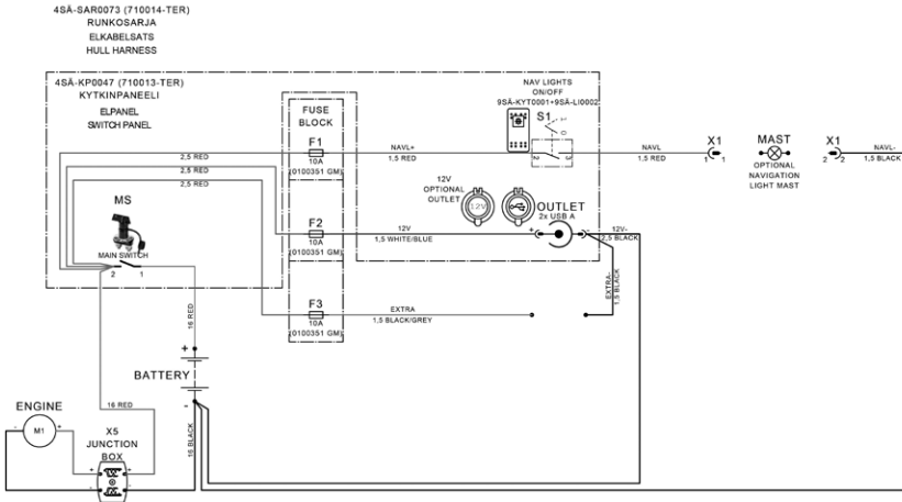
Abb. 11. Schaltplan für Terhi 400 CC
