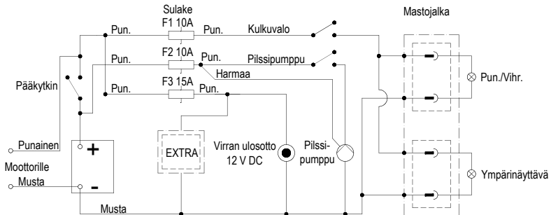
Kuva 10. Terhi 480 BR, 480 Sport -kytentaavaio
