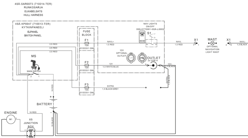
Bild 11. Kopplingsschema för Terhi 400 CC
